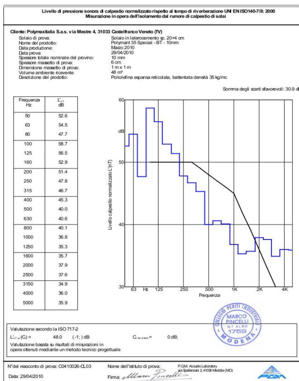
Grafico 2: Certificato di prova Polymant 35 Special BT Sp. 10mm con massetto sp. 6 cm P.G.M. di P.I. Marco Pincelli via Spallanzani, 2 41036 Medolla (MO)
