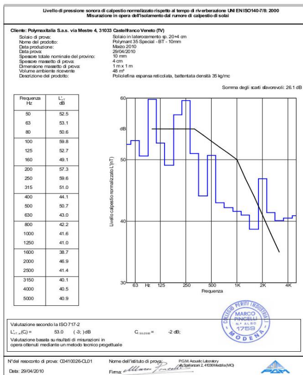
Grafico 1: Certificato di prova Polymant 35 Special BT Sp. 10mm con massetto sp. 4 cm P.G.M. di P.I. Marco Pincelli via Spallanzani, 2 41036 Medolla (MO)
