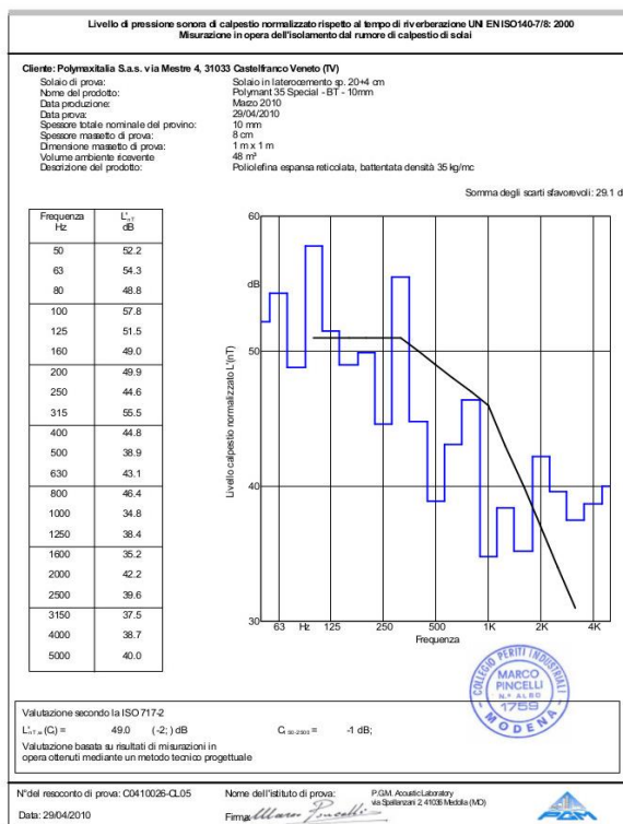
Grafico 3: Certificato di prova Polymant 35 Special BT Sp. 10mm con massetto sp. 8 cm P.G.M. di P.I. Marco Pincelli via Spallanzani, 2 41036 Medolla (MO)
