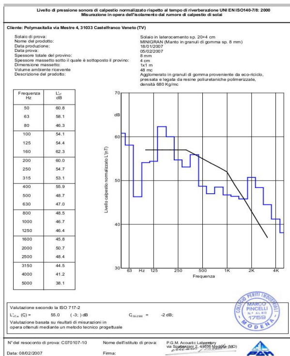
Grafico 4: L tot,w MINIGRAN sp. 8 mm - massetto sp. 4 cm
