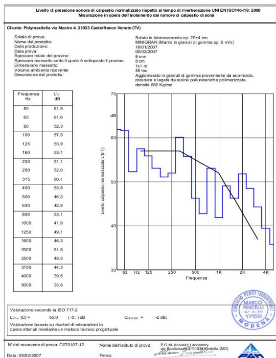
Grafico 6: L tot,w MINIGRAN sp. 8 mm - massetto sp. 8 cm
