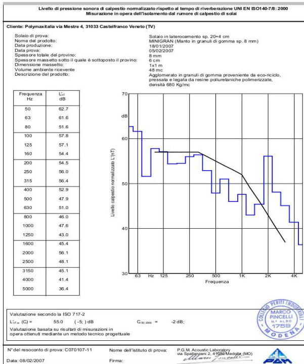
Grafico 5: L tot,w MINIGRAN sp. 8 mm - massetto sp. 6 cm
